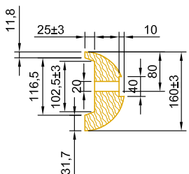
D-D (2:1)
